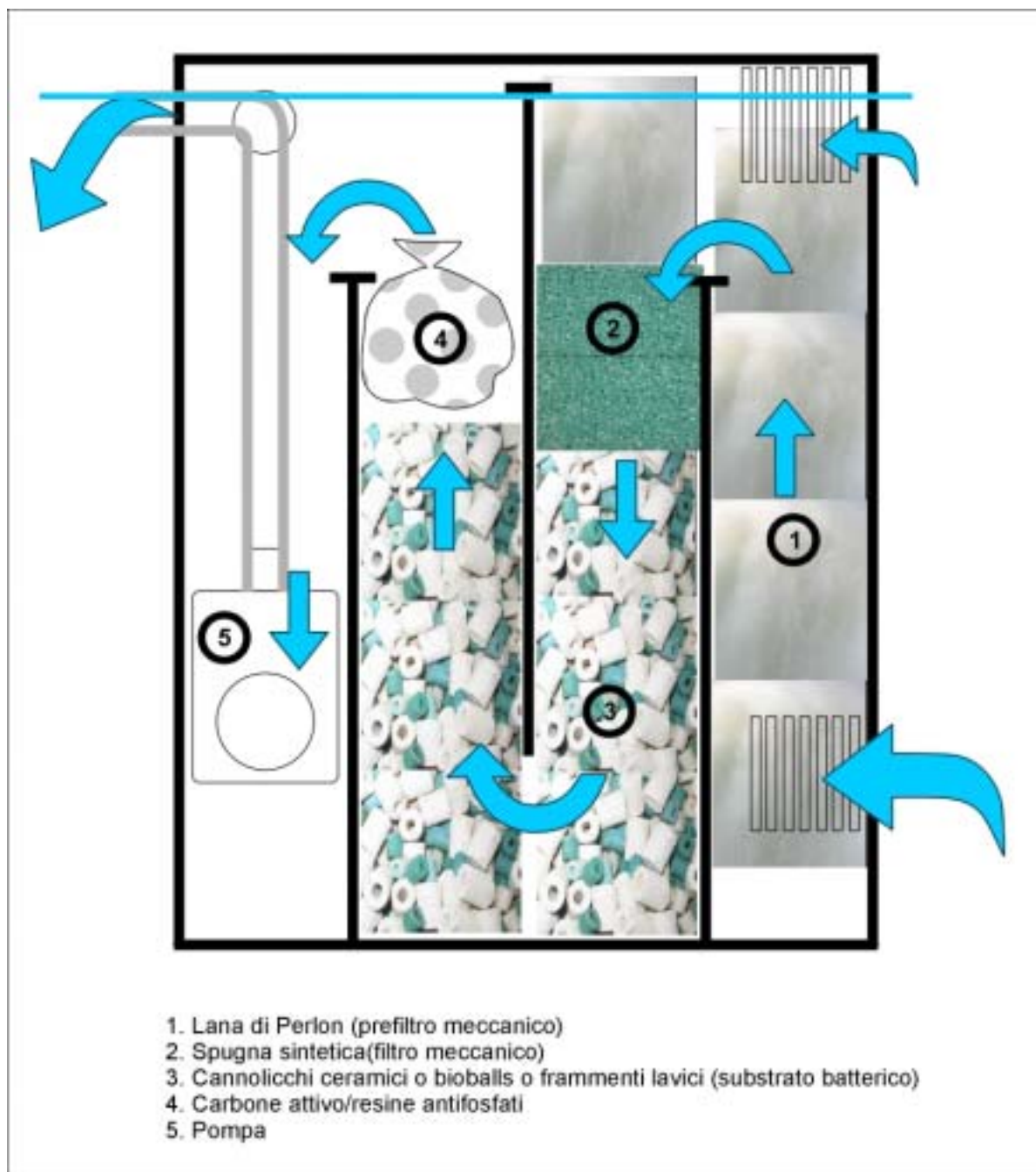
Schema di filtro biologico a comparti
